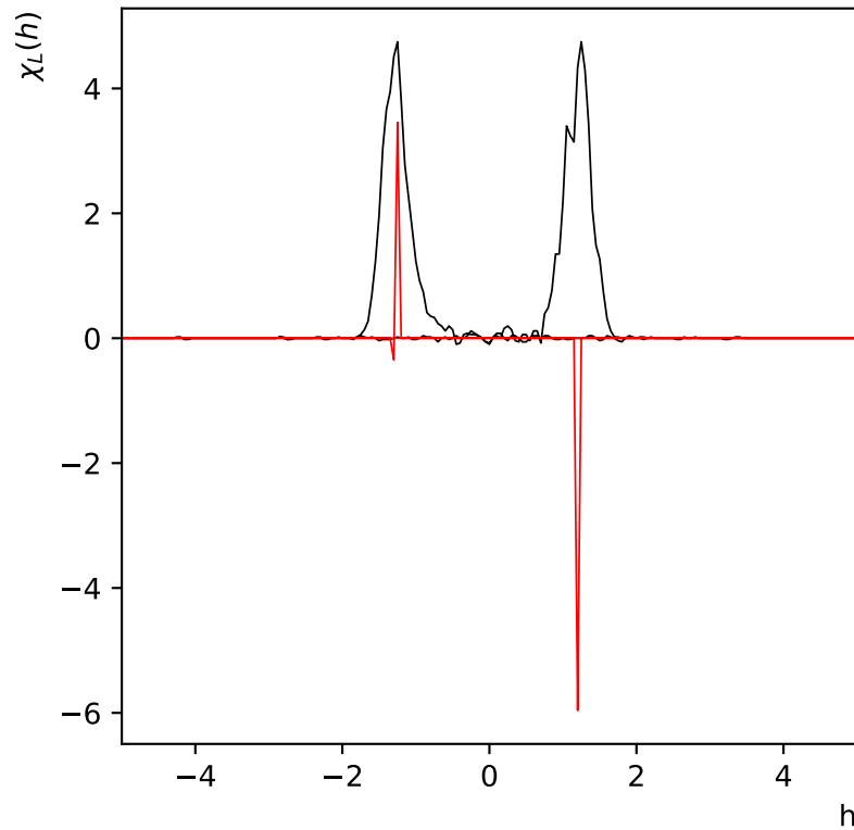
\chi_L(h) réseau de taille L=32 à T=1.5
