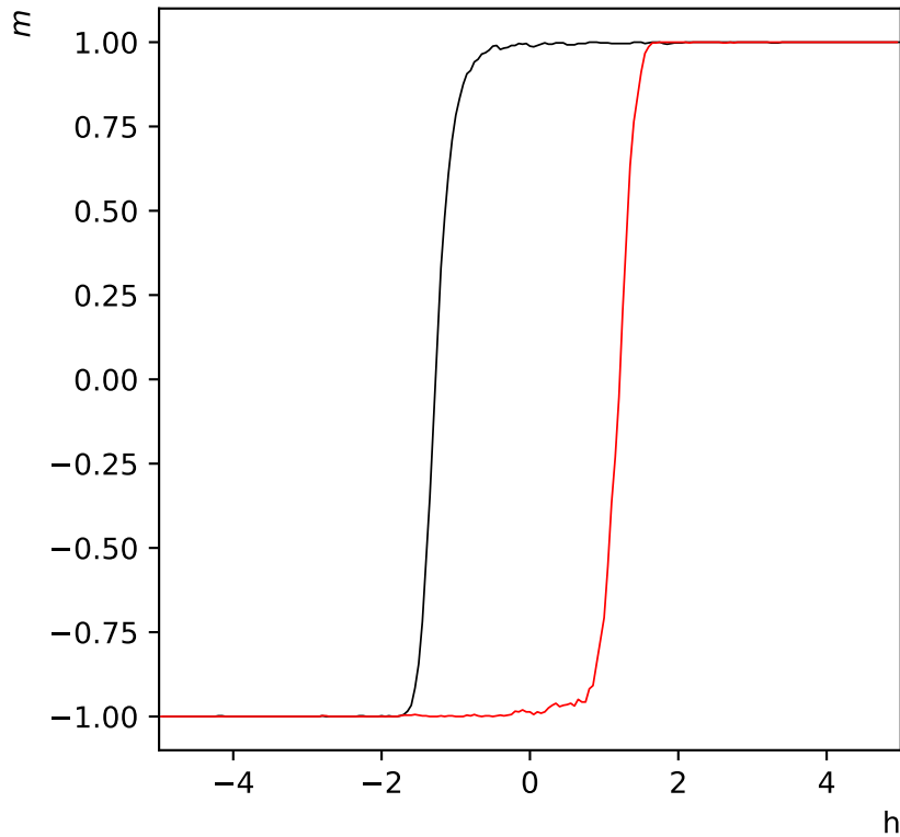
Hystérésis de l'aimantation réseau de taille L=32 - h=5 à T=1.5
